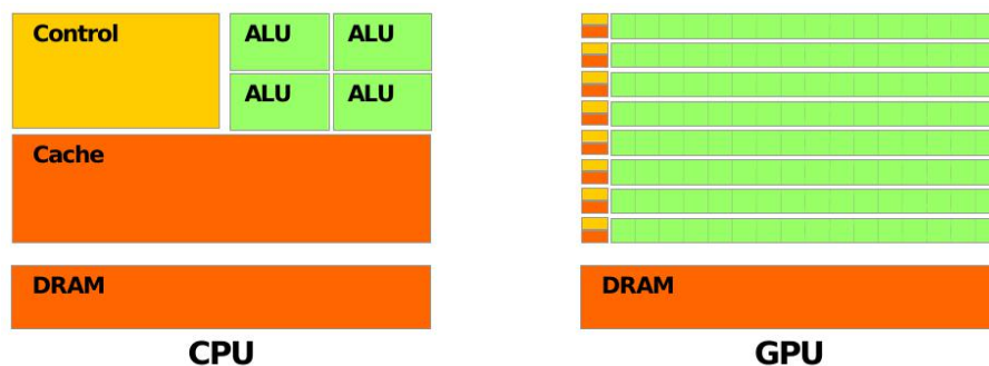
Abbildung 2.7: Architektur einer Multicore-CPU und einer GPU [NVIDIA]
