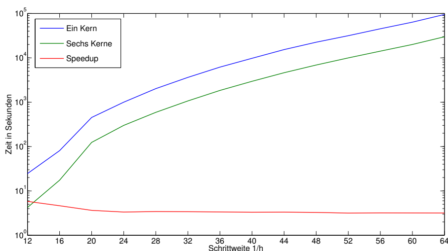
Abbildung 4.13: Zeitmessungen der seriellen Laufzeit gegen OpenMP Parallelisierung
