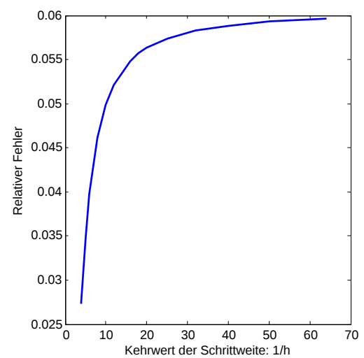
(b) Entwicklung des relativen Fehlers zur exakten Referenzlösung (bezüglich der Euklidischen Norm)
