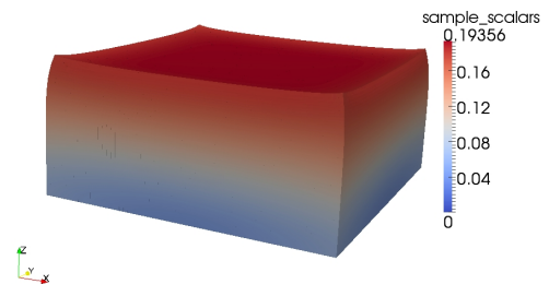
(f) Näherungslösung zu h = \frac{1}{64}
