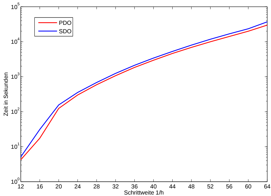
Abbildung 4.15: Zeitvergleich CPU
