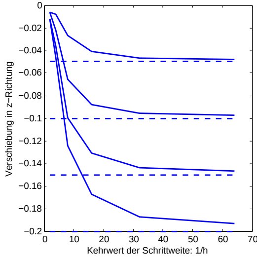
Abbildung 4.7: Verschiebungen entlang der z -Achse in den Gitterpunkten (0.5, 0.5, 0.25) , (0.5, 0.5, 0.5) , (0.5, 0.5, 0.75) und (0.5, 0.5, 1) (von oben nach unten) zu verschiedenen Schrittweiten h . Gestrichelt sind die Werte gekennzeichnet, die das Hookesche Gesetz an diesen Stellen vorhersagt.
