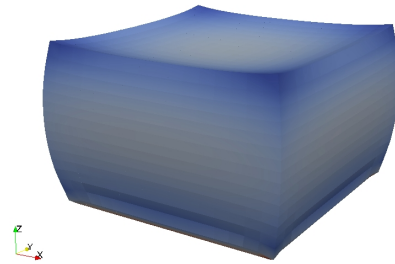
(d) Lösung der Penalty-Methode zu h = \frac{1}{16}
