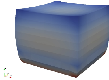
(b) Lösung der Penalty-Methode zu h = \frac{1}{8}
