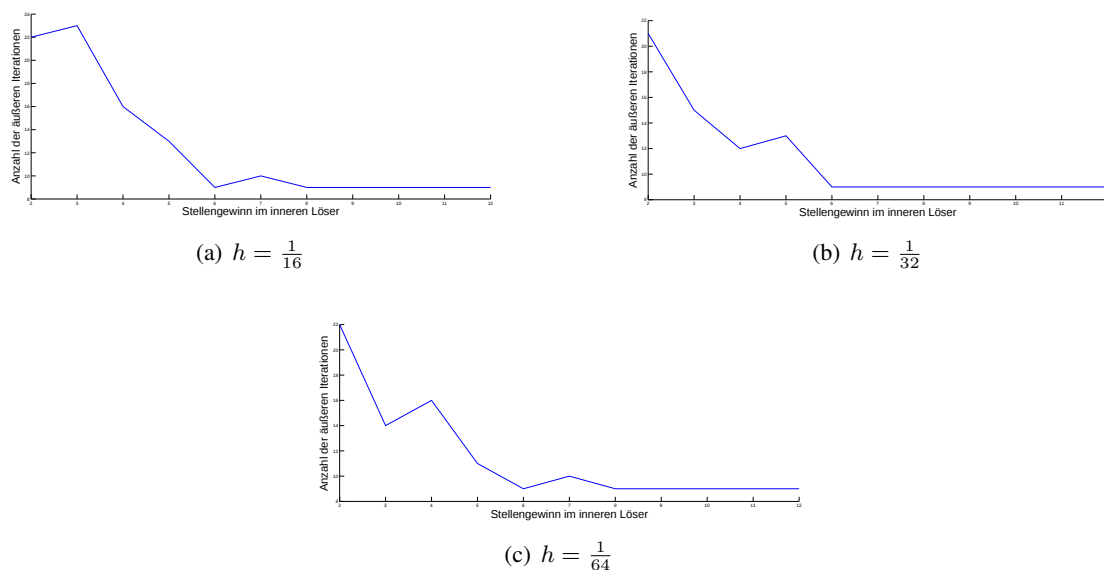
Abbildung 4.19: Gesamtzahl der äußeren Iterationen zu verschiedenen Schrittweiten h
