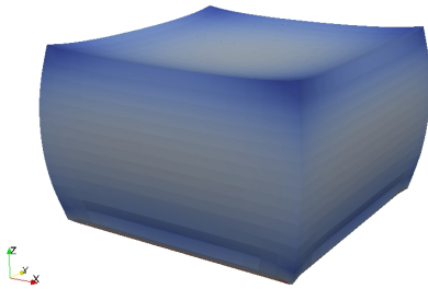
(c) Lösung bei semi-impliziter Integration zu h = \frac{1}{16}
