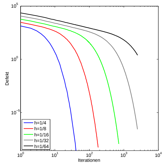
(b) Richardson mit Gauß-Seidel-Vorkonditionierung
