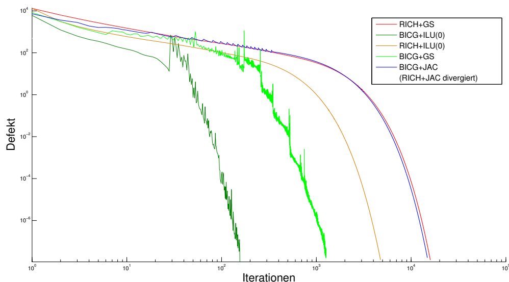
Abbildung 4.22: Konvergenzverlauf bei h = \frac{1}{32}
