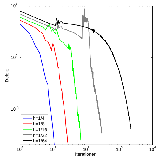
(d) BiCGStab mit Gauß-Seidel-Vorkonditionierung
