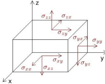
Abbildung 2.1: Dreidimensionaler Spannungszustand
