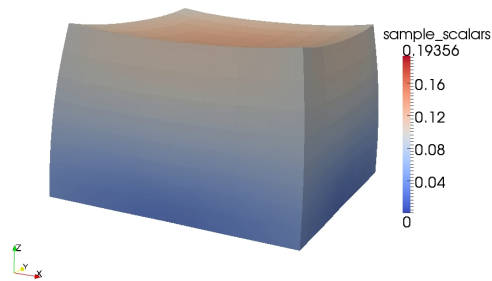
(c) Näherungslösung zu h = \frac{1}{8}
