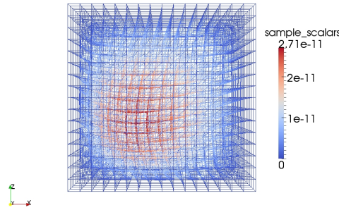
Abbildung 4.1: Analytische Referenzlösung ausgewertet auf einem Gitter der Schrittweite h = \frac{1}{16}
