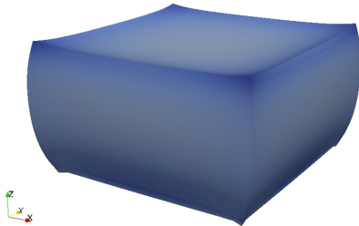
(e) Lösung bei semi-impliziter Integration zu h = \frac{1}{32}
