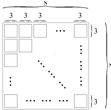
Abbildung 2.5: Blockstruktur der Matrix beim Ordnen nach Knoten
