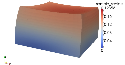
(d) Näherungslösung zu h = \frac{1}{16}
