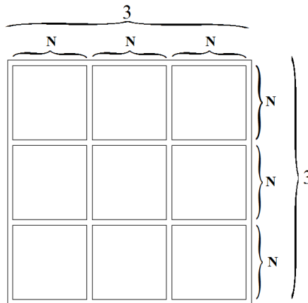
Abbildung 2.6: Blockstruktur der Matrix beim Ordnen nach Kopplung
