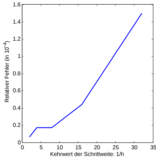
Abbildung 4.9: Verhalten des relativen Fehlers e = \frac{\|u_{\text{Penalty}} - u_{\text{Semi-implizit}}\|_2}{\|u_{\text{Semi-implizit}}\|_2} zwischen den Näherungslösungen des Penalty-Verfahrens und der semi-impliziten Integrationsmethode der Randbedingungen.
