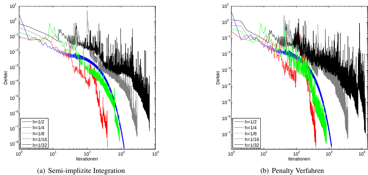
Abbildung 4.11: Konvergenzverhalten bei Verwendung der beiden Integrationsmethoden. Simuliert wurde die oben beschriebene Problemsituation unter Verwendung der Schrittweiten \frac{1}{2} , \frac{1}{4} , \frac{1}{8} , \frac{1}{16} und \frac{1}{32} . Es ist deutlich zu erkennen, dass sich bei der Verwendung des Penalty-Verfahrens mehr Instabilitäten ergeben als bei der semi-impliziten Integrationsmethode. Restarts erfolgten hier bei schlecht konditionierten Divisionen, das heißt in dem Fall „Divisor < Divident \cdot 10^{-14} “.
