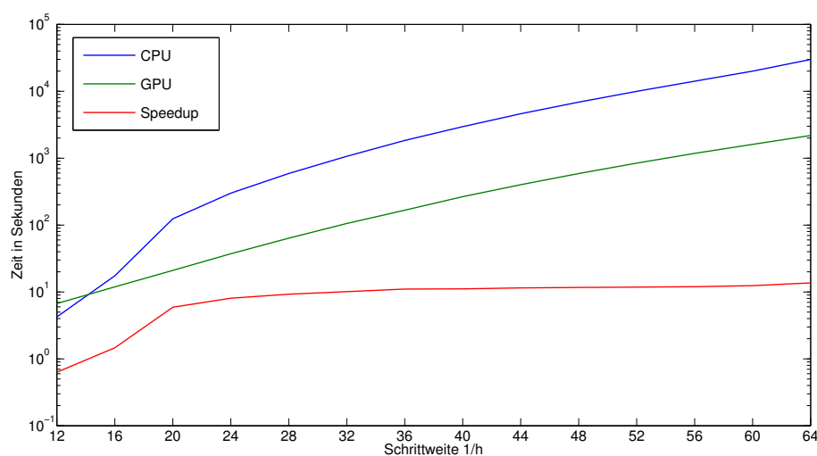
Abbildung 4.14: Laufzeitvergleich von CPU und GPU
