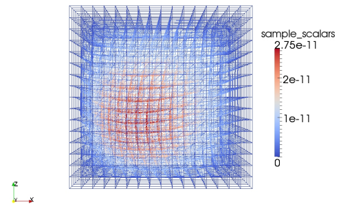
(d) Näherungslösung zu h = \frac{1}{16}
