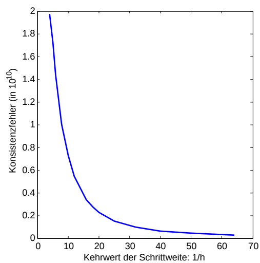
(a) Asymptotisches Verhalten des Konsistenzfehlers
