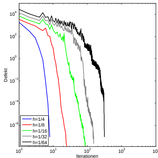
(c) BiCGStab mit Jacobi-Vorkonditionierung
