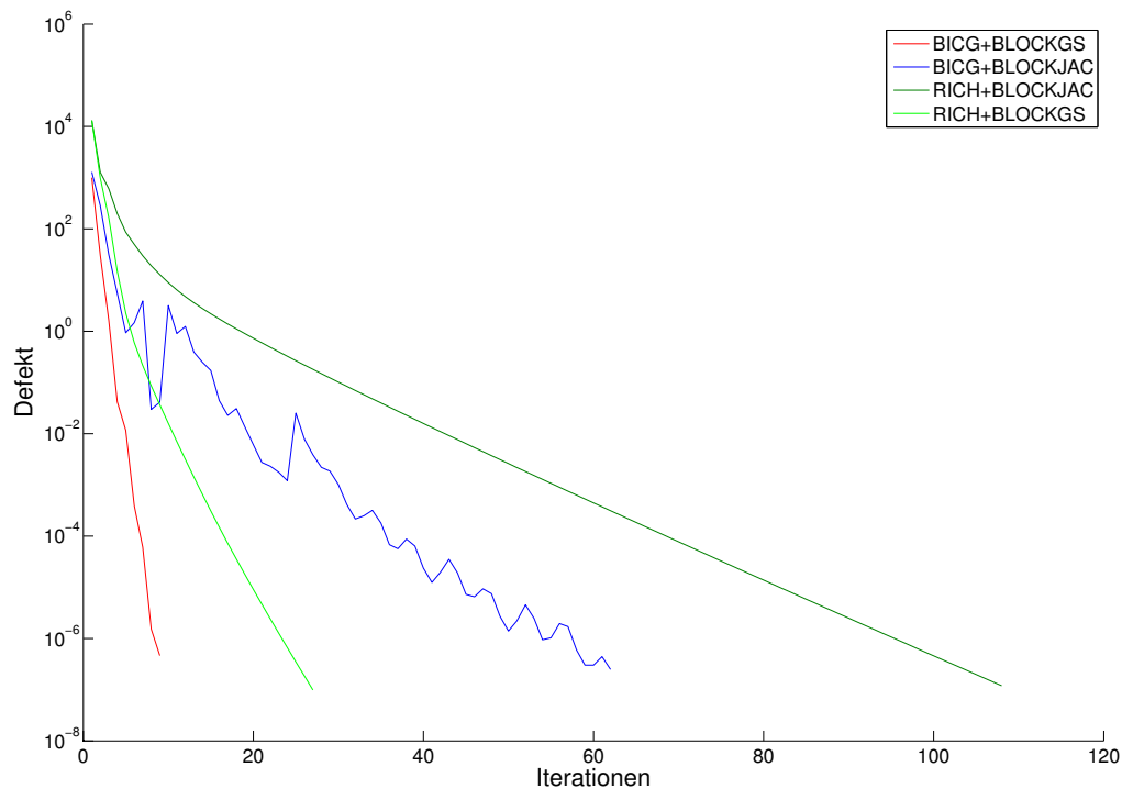
Abbildung 4.18: Konvergenzverlauf mit h = \frac{1}{32}
