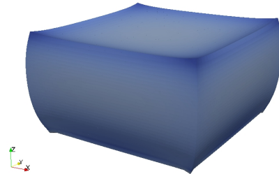
(f) Lösung der Penalty-Methode zu h = \frac{1}{32}
