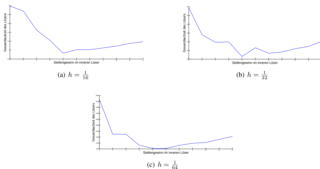
Abbildung 4.21: Gesamtrechendauer zu verschiedenen Schrittweiten h
