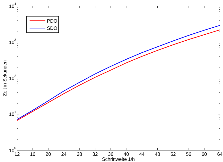
Abbildung 4.16: Zeitvergleich GPU
