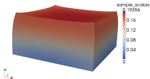
(e) Näherungslösung zu h = \frac{1}{32}
