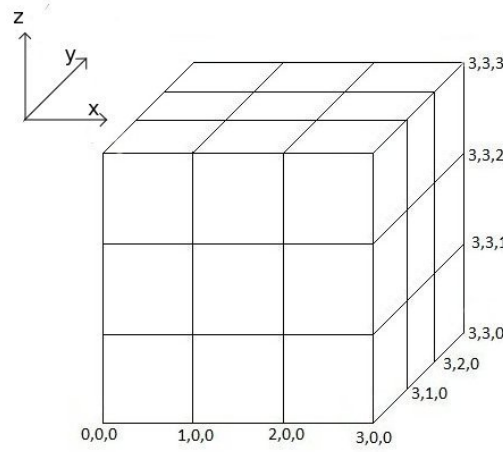
Abbildung 2.3: [0, 1]^3 äquidistant zerlegt
