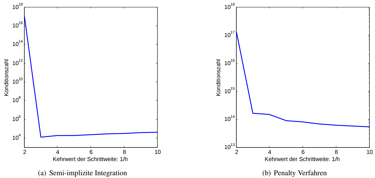
Abbildung 4.10: Entwicklung der Konditionszahl der Systemmatrix bei Verwendung der beiden Integrationsmethoden. Man beachte die äußerst schlechte Kondition bei h = \frac{1}{2} , die durch die entartete Kopplungssituation bei Verwendung der einseitigen Differenzenquotienten auf einem 3 \times 3 \times 3 -Gitter entsteht (siehe Kapitel 2.2).
