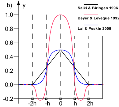
Abbildung 2.4: Verschiedene Lastdistributionsfunktionen nach [Mittal]
