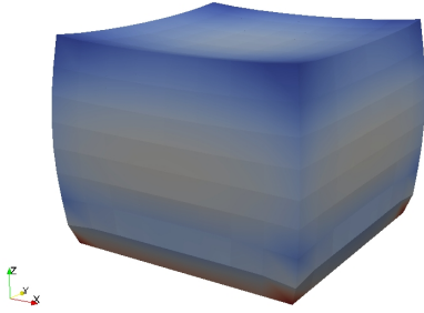
(a) Lösung bei semi-impliziter Integration zu h = \frac{1}{8}
