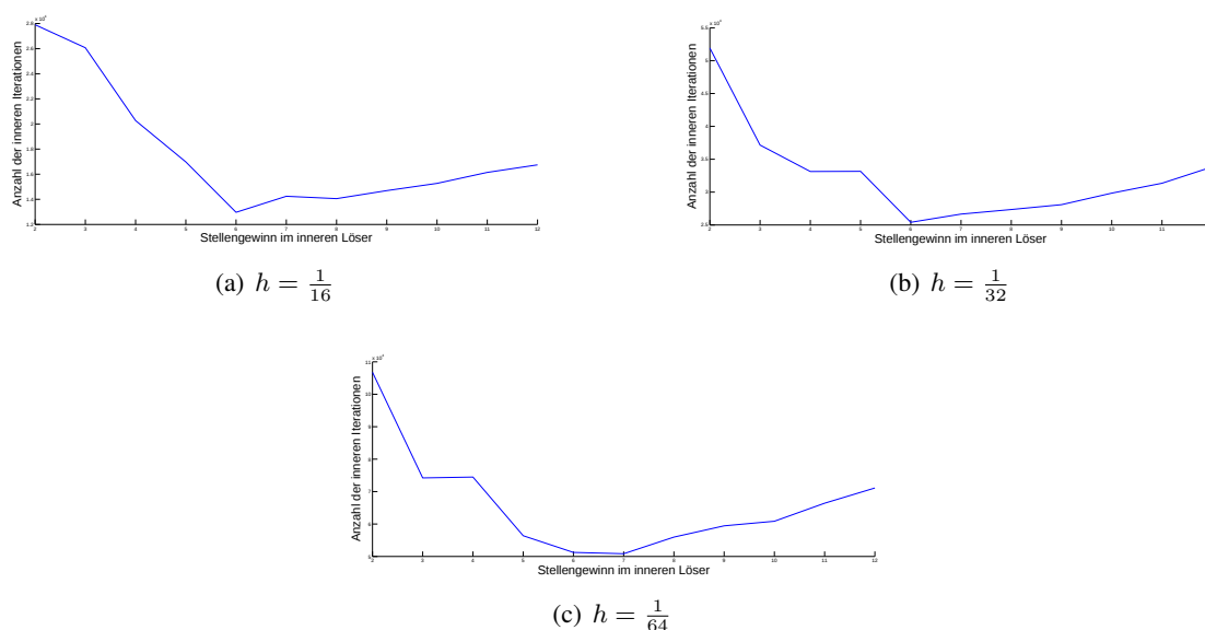
Abbildung 4.20: Gesamtzahl der inneren Iterationen zu verschiedenen Schrittweiten h
