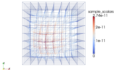
(c) Näherungslösung zu h = \frac{1}{8}
