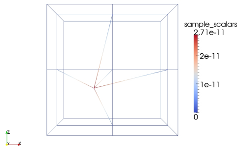
(a) Näherungslösung zu h = \frac{1}{2}
