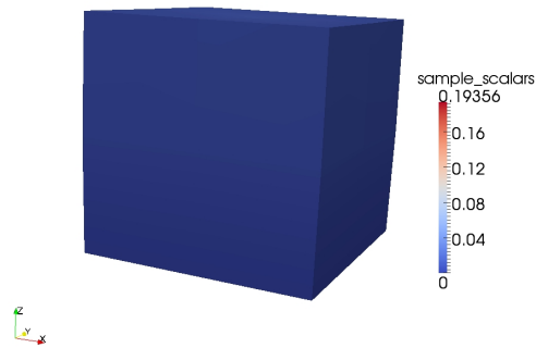
(a) Näherungslösung zu h = \frac{1}{2}
