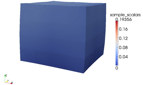
(b) Näherungslösung zu h = \frac{1}{4}
