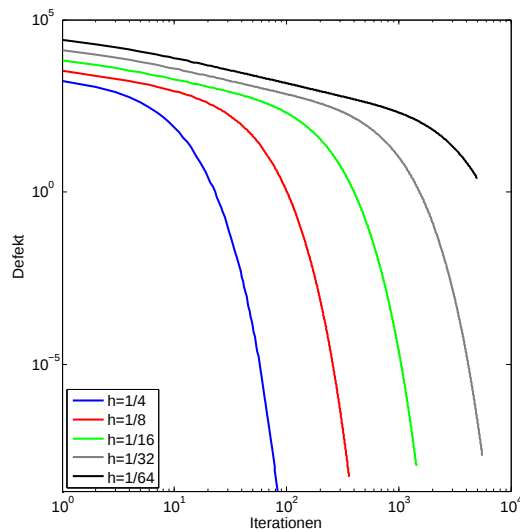
(a) Richardson mit Jacobi-Vorkonditionierung
